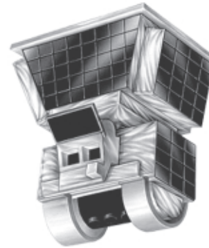
CERES
