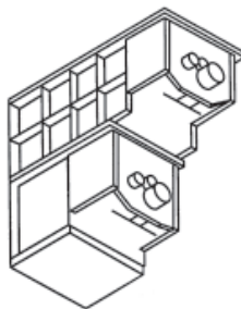
AMSU-A
